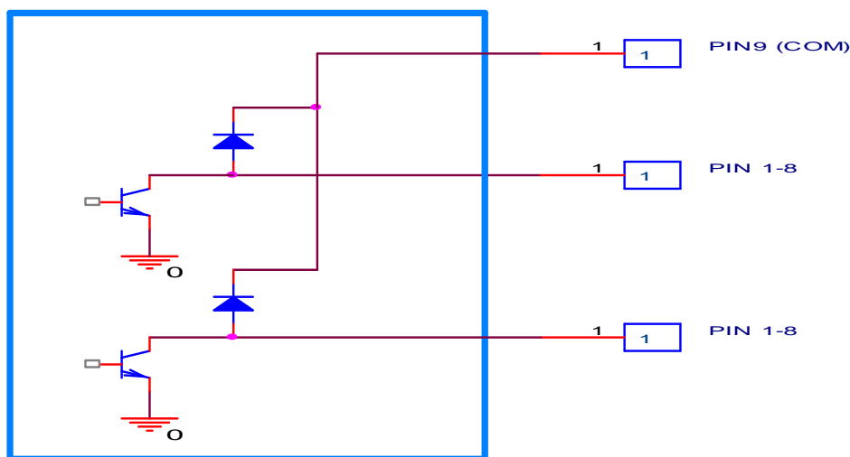
Schema internă a 2 din cele 8 ieșiri fig.2
